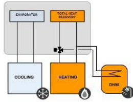
VACSR (4 - pipes)
