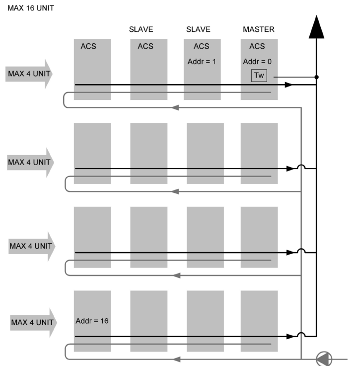
Anschlusschema für modulares System - Adressierung
