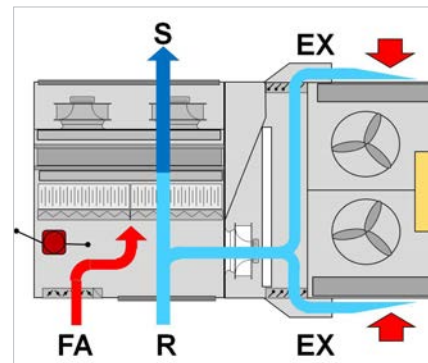
Il dispositivo di controllo della pressione ambiente è fornito di serie nell'unità in configurazione con estrazione ed espulsione (sigla Clivet di riferimento CCK o CCKP)
