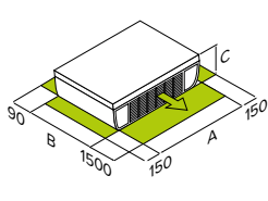
CFF / CFFA CAS Unité visible
