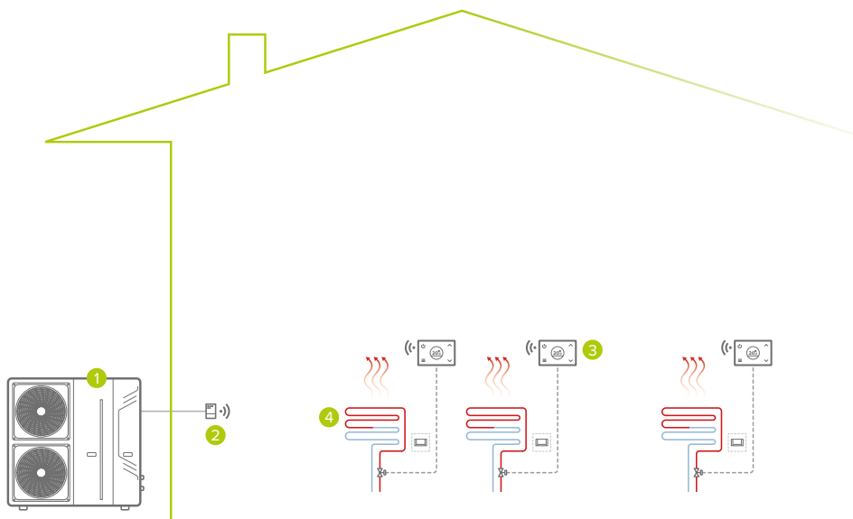
Installation à zone unique seulement chaud, radiante/unités terminales, connexion via Wi-Fi au générateur et via câble à la distribution
