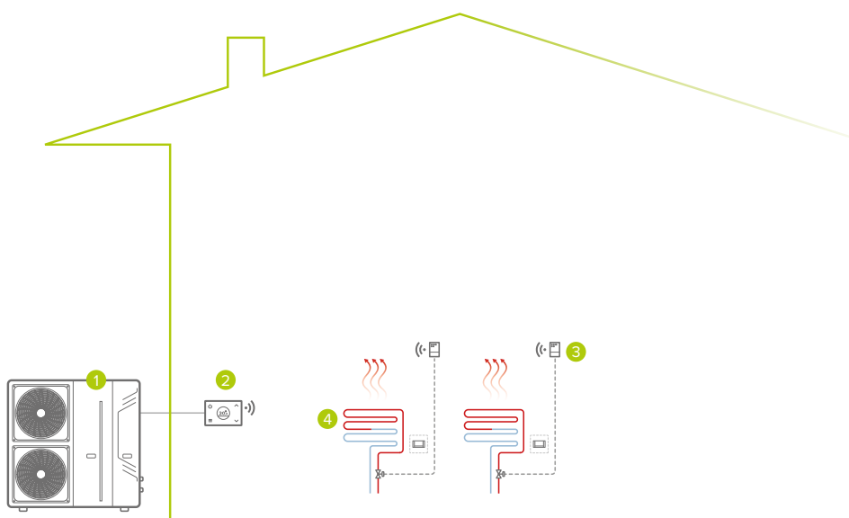
Installation à zone unique seulement chaud, radiante/unités terminales, connexion via câble au générateur et Wi-Fi à la distribution
