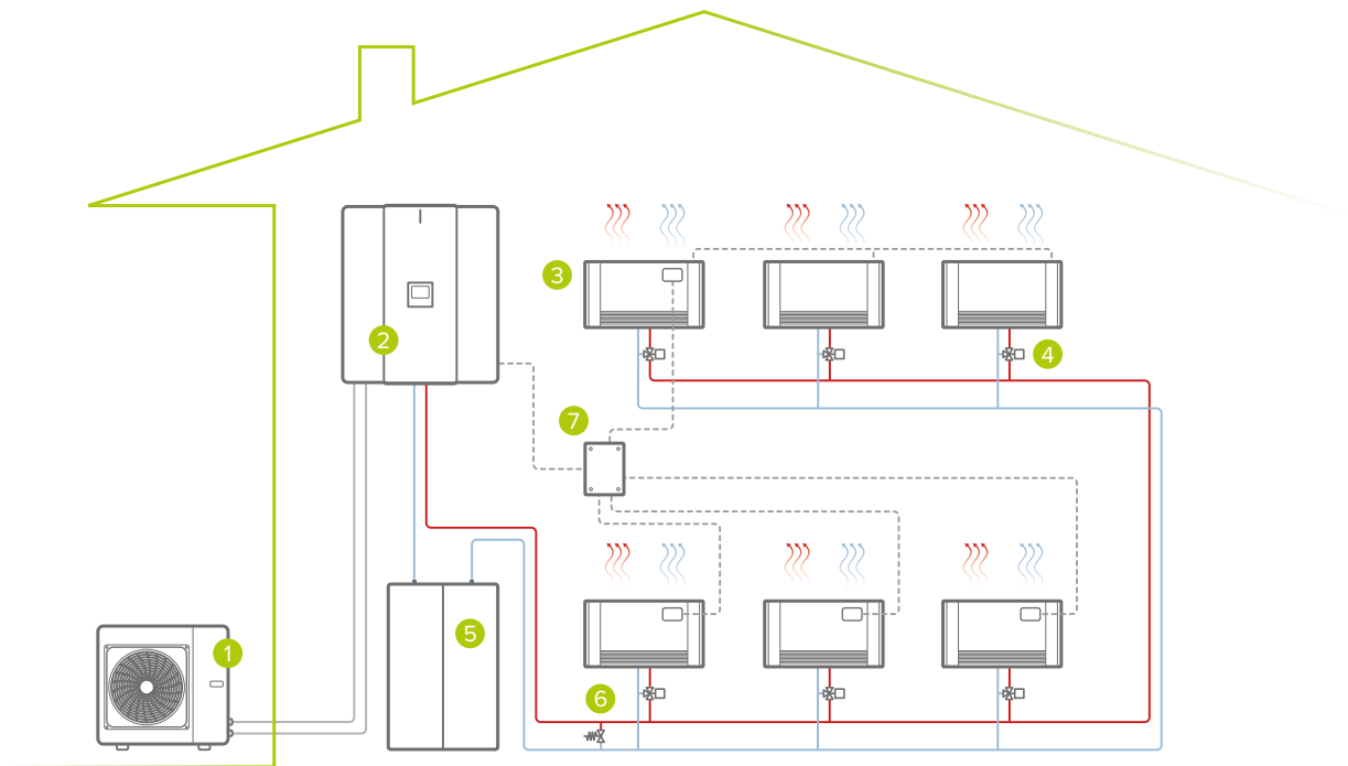
Système à zone unique: chauffage/refroidissement
