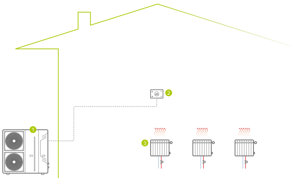
Installation à zone unique, radiateurs, connexion via câble au générateur
