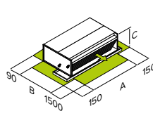
CFF / CFFA UNC Unité intégrée
