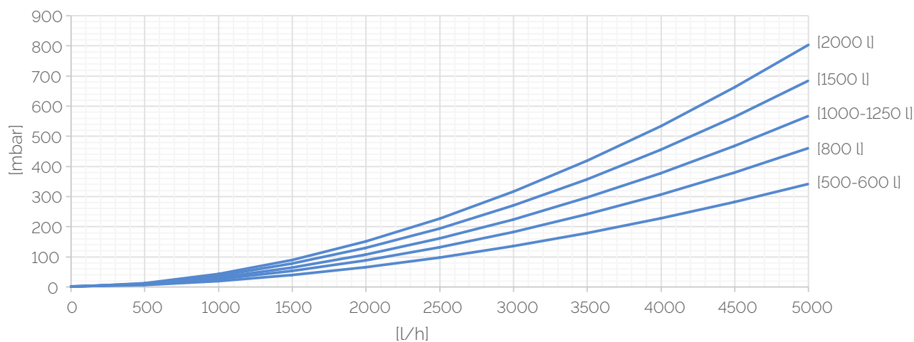
Druckverluste des unten Wärmetauschers
