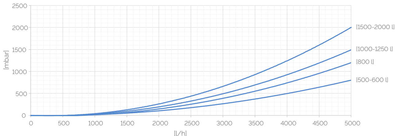
Druckverluste des TWW Wärmetauschers
