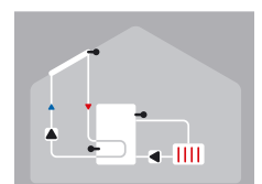
Solarthermie mit Kühlung 3 (Kühlung des Speichers)
