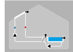
Solarthermie mit Wärmetauscher (Sensor am Sekundärkreislauf) und Schwimmbad
