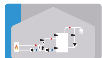
Speicherladung mit VFS, Pumpe am Primärkreislauf, Legionellenschutz und Zirkulationspumpe
