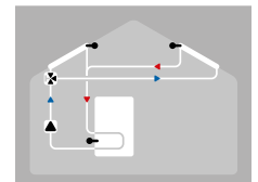
Solarthermie mit 2 Kollektoren
