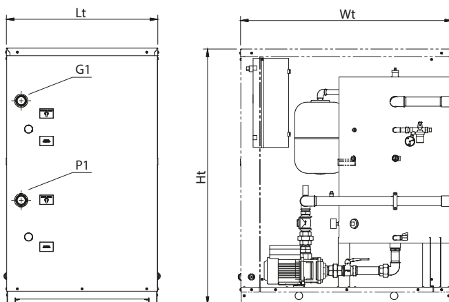
Abmessungen HPT; stehende Ausführung
