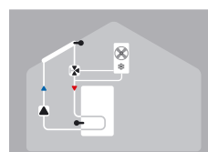
Solarthermie mit Kühlung 1 (Kühlung des Speichers)
