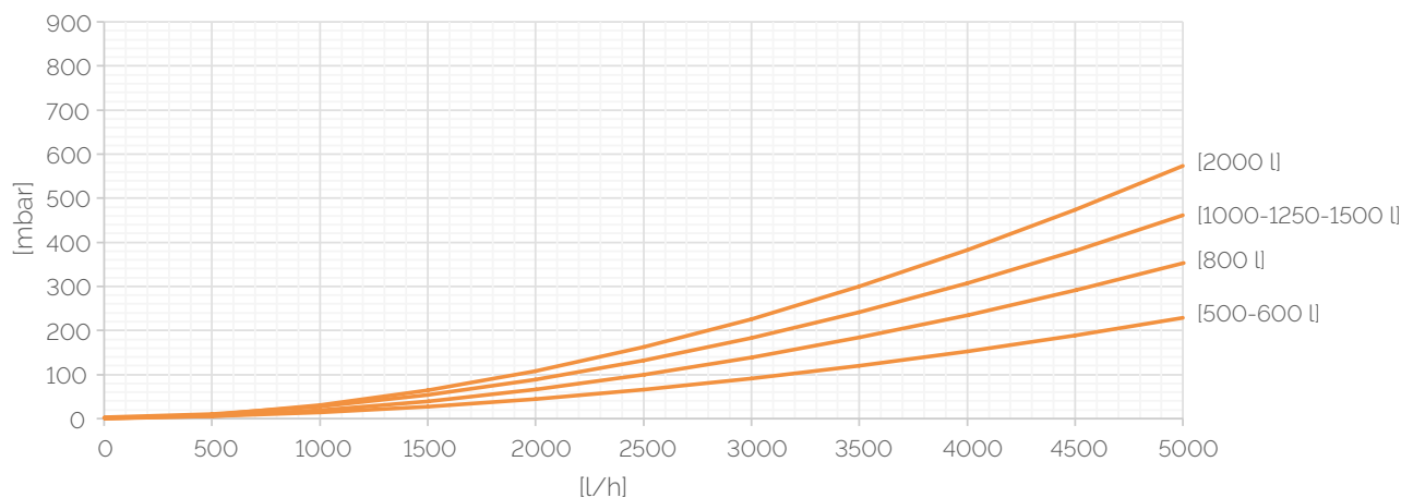
Druckverluste des oben Wärmetauschers
