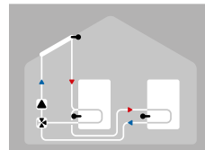
Solarthermie mit 2 Speichern und Ventil
