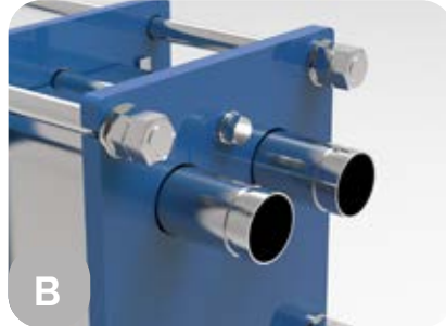
B Victaulic-Anschluss
