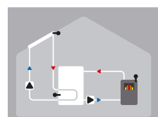
Solarthermie mit Holzheizkessel
