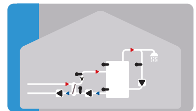
Speicherladung mit VFS, Pumpe am Primär- und TWW-Kreislauf
