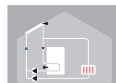
Solarthermie mit Kühlung 2 (Kühlung des Speichers)
