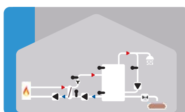
Speicherladung mit VFS, Pumpe am Primärkreislauf, Legionellenschutz und Sedimentabfluss
