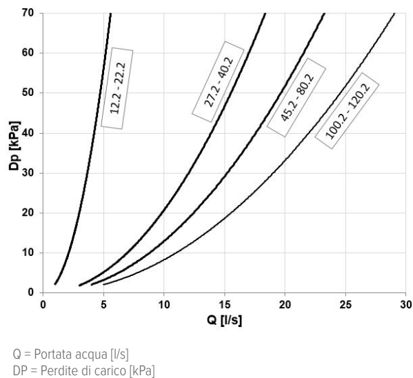
Perdite di carico valvola 3 vie modulante (VS3MHX - VS3MCX)
