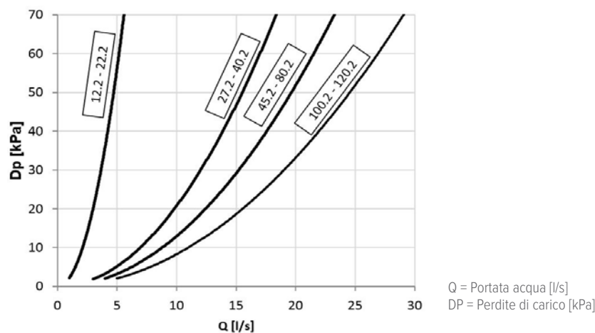
Perdite di carico valvola deviatrice ACS
