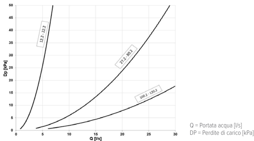
Perdite di carico filtro a maglia d'acciaio
