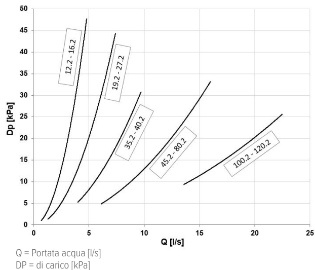
Perdite di carico valvola 2 vie modulante (VS2MHX - VS2MCX)
