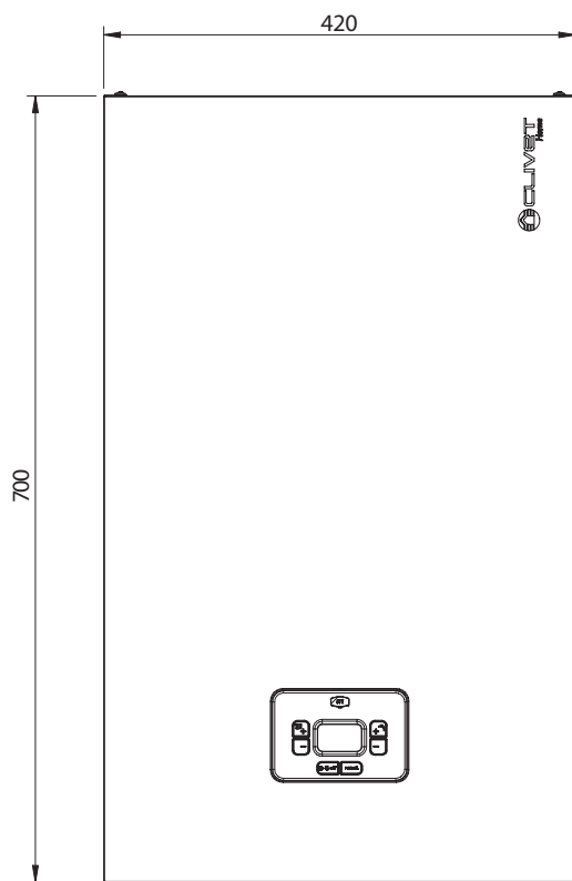
Vista frontale
