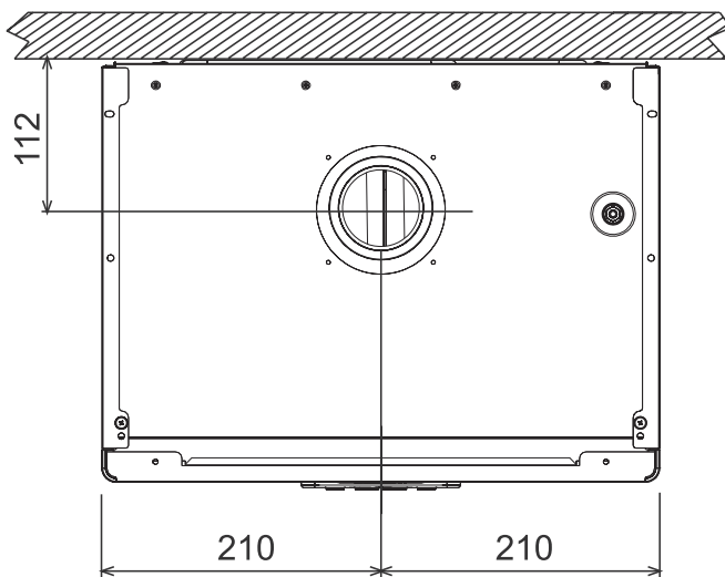
Vista dall'alto
