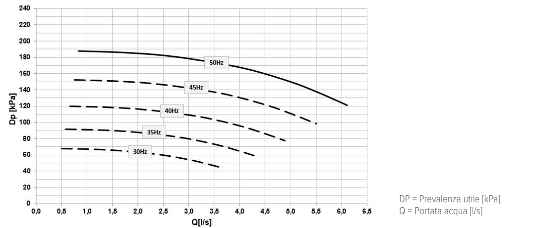
Curva prevalenza pompe grandezze 25.2 - 30.2 - 35.2
