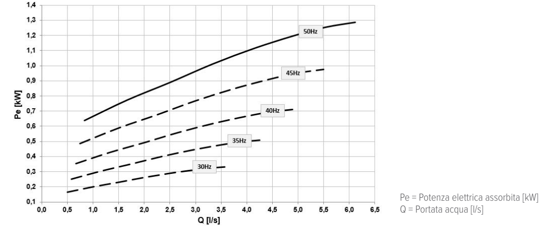
Curva assorbimento pompe grandezze 25.2 - 30.2 - 35.2
