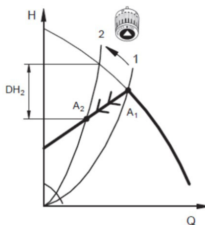
Regelung mit Pumpe mit proportionaler Förderhöhe Die Förderhöhe wird um DH_2 reduziert
